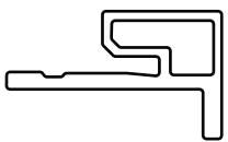
Bordure de finition UH59
